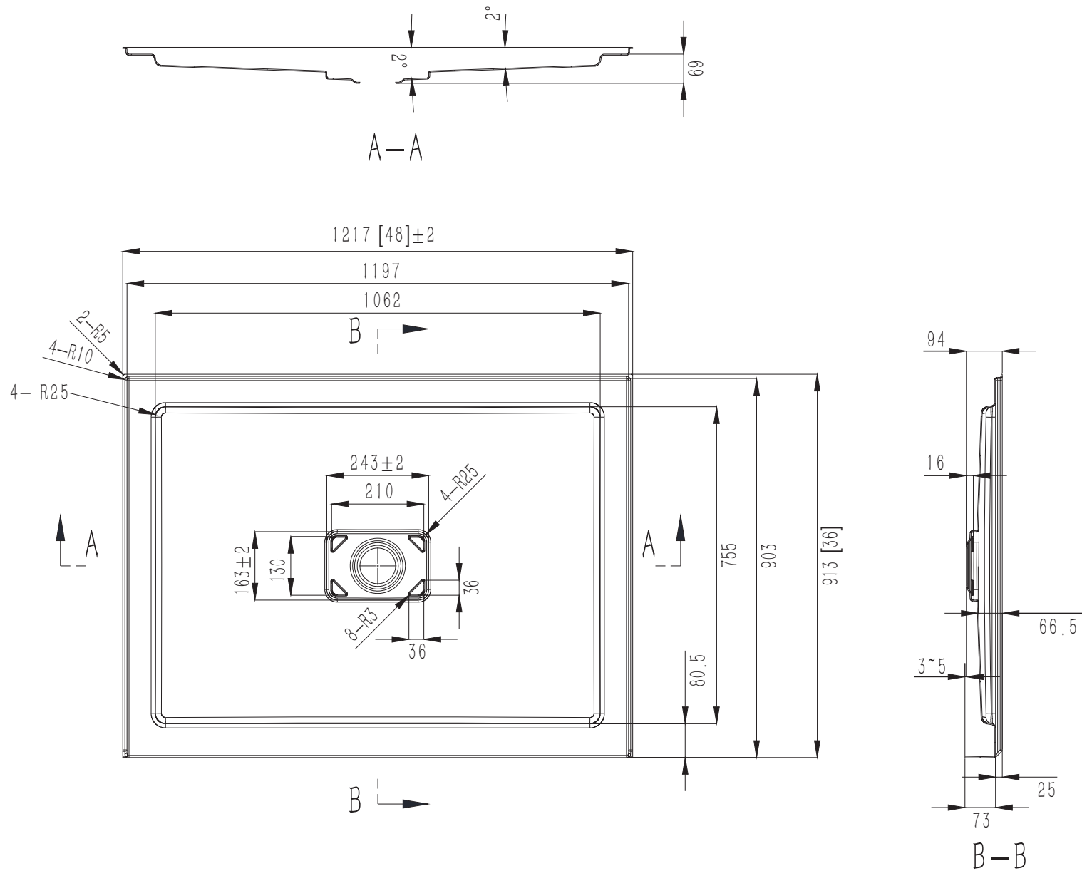
Base de douche 48"x36"
